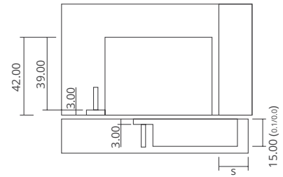
HINGES
